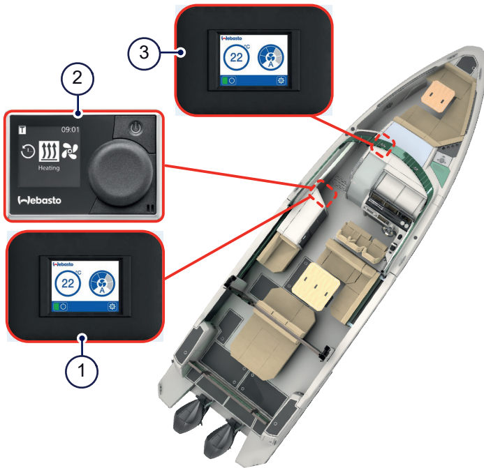
Kuva 4.18 - Lämpötilan ohjauspaneeli
