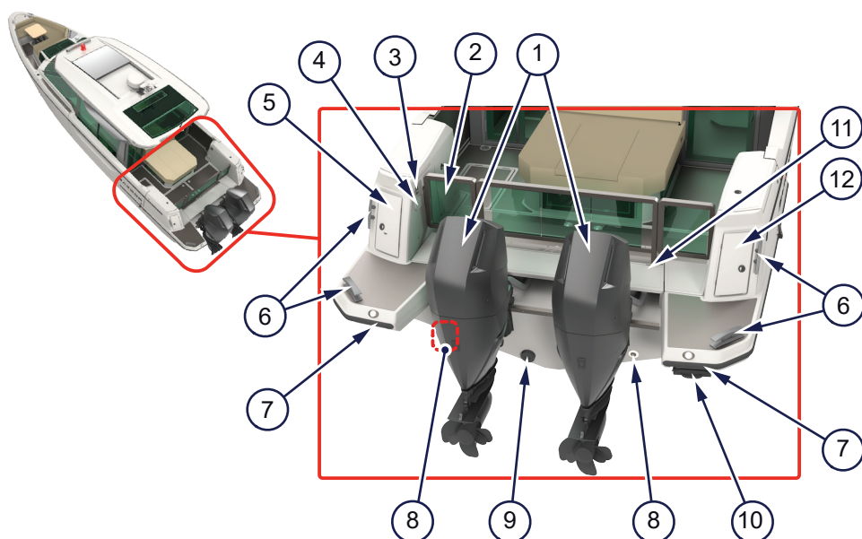
Kuva 4.7 - Uimatasanne
