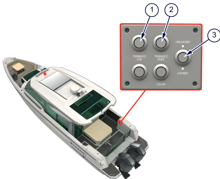
Kuva 4.13 - Sivuterassin ohjauspaneeli
