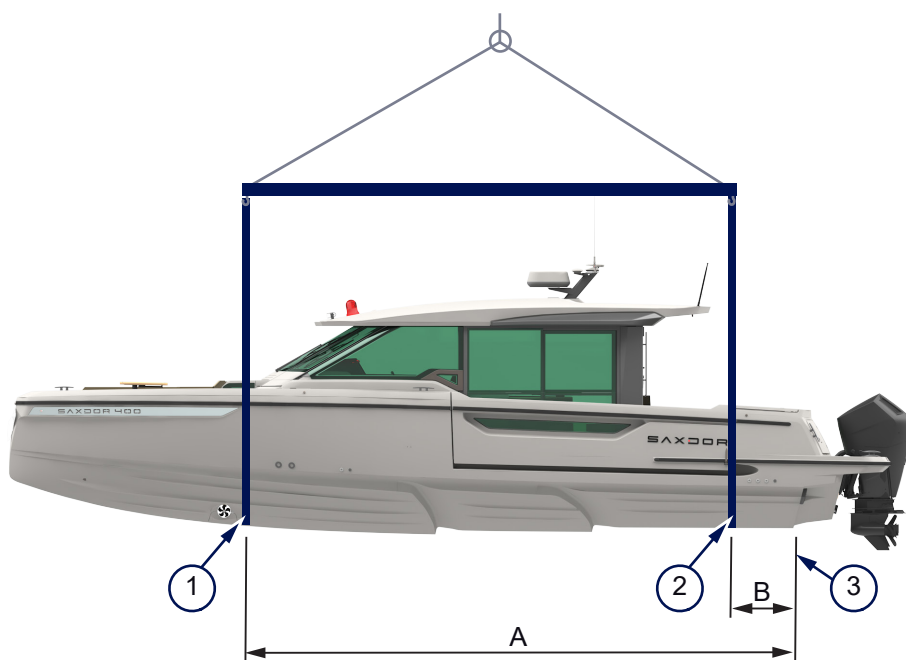
Kuva 4.23 - Nostopisteet
