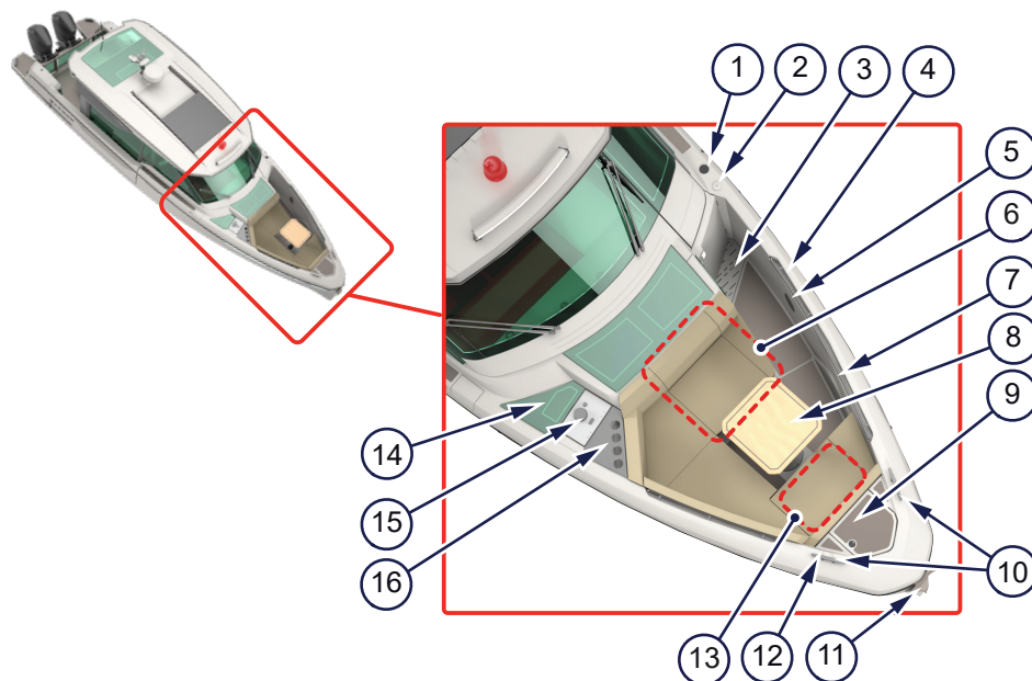
Kuva 4.2 - Etukansi
